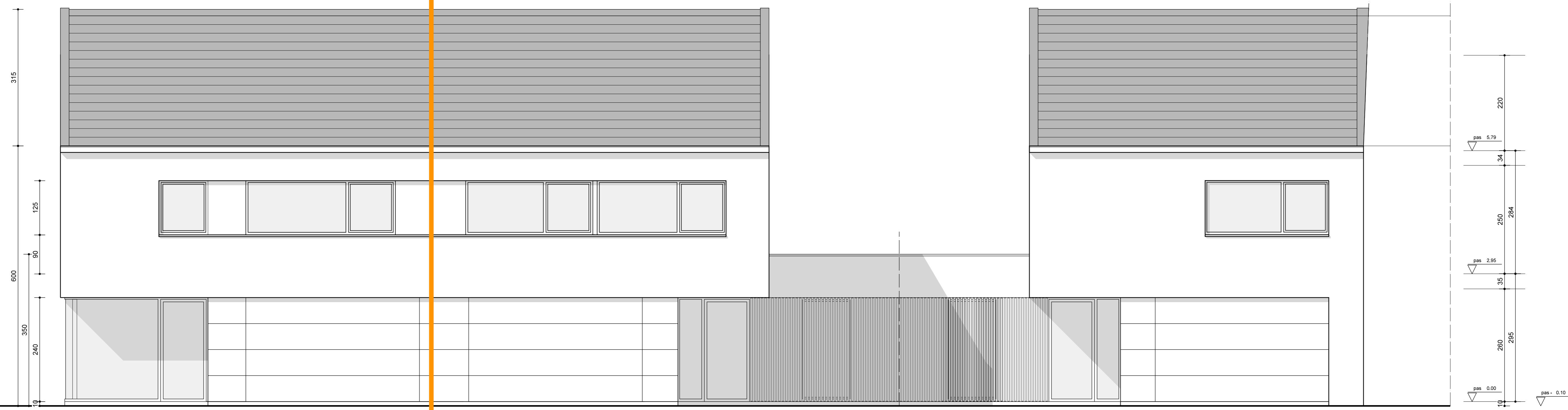
VOORGEVEL
