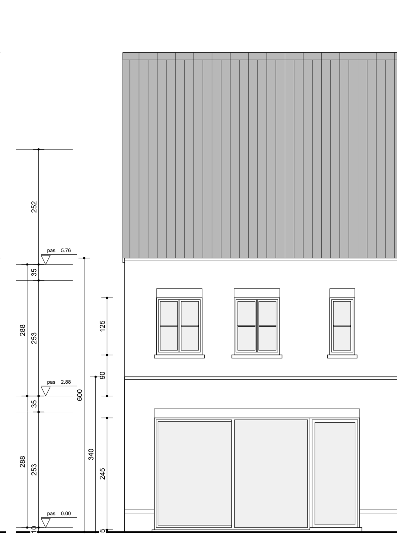
ACHTERGEVEL
