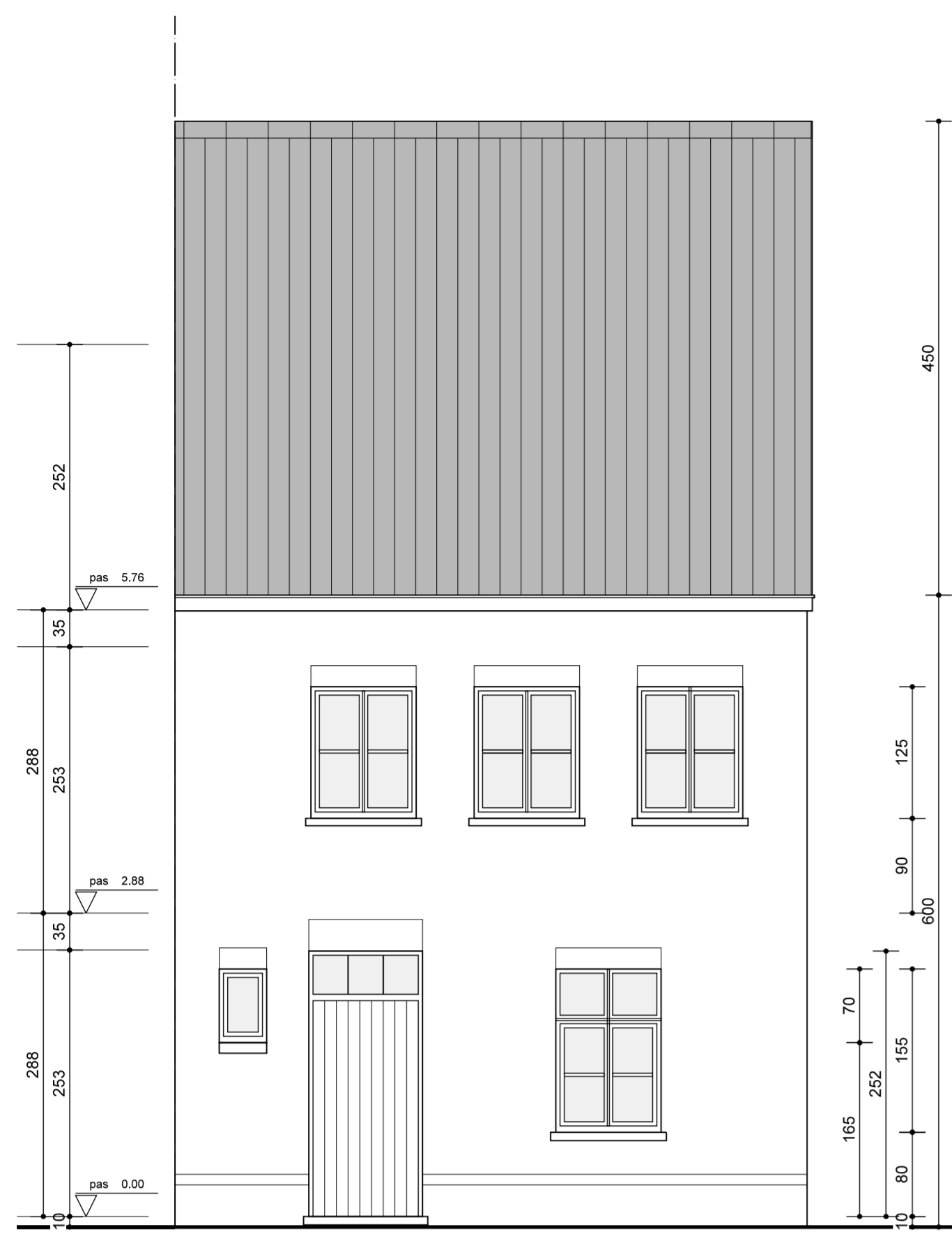
VOORGEVEL
